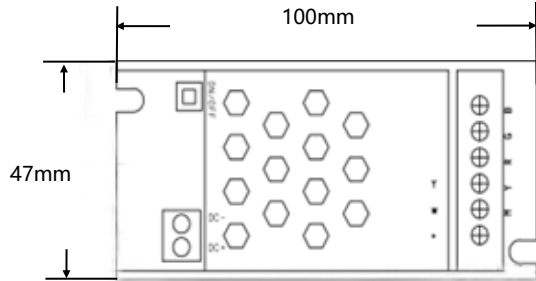
正面图
