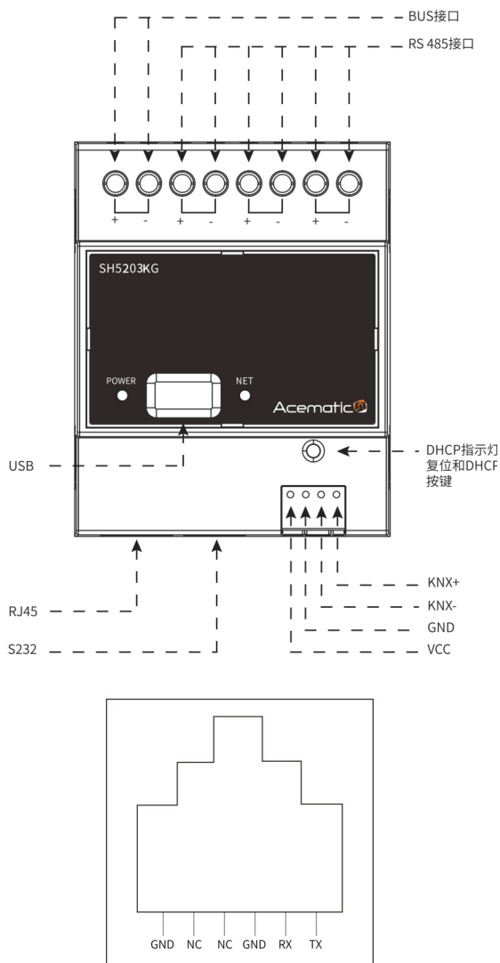
RS232接口定义
