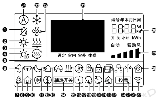
图3.2 线控器液晶图示
