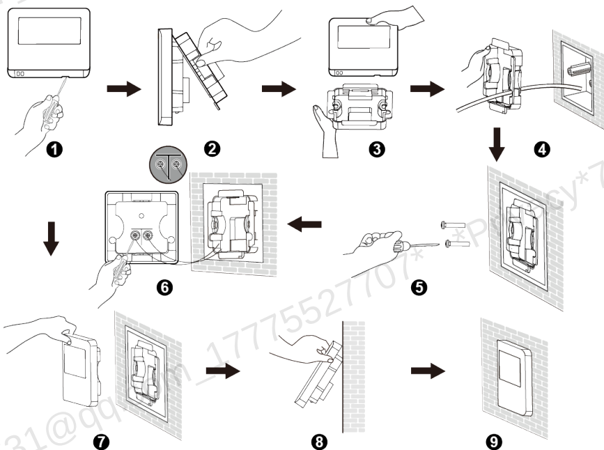
图5.10 线控器安装示意图
