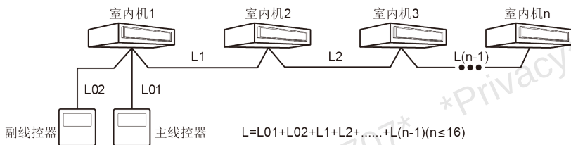
图 5.3 通讯线长度
