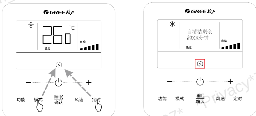
图6.7 自清洁状态显示
