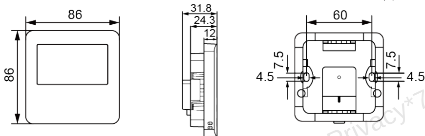
图5.1 线控器尺寸
