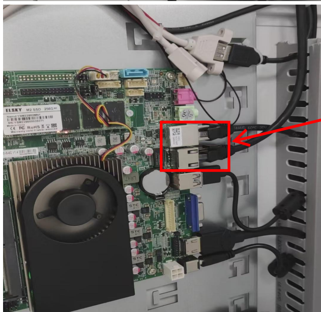
钣金电脑网络接口*2
